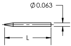
T (TUNGSTEN P/N: 635-063-SERIES)
