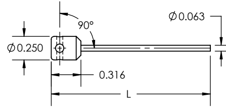
H-90 (TUNGSTEN HOLDER ASSEMBLY 90 DEG P/N: 002-0771)
