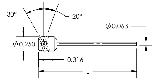
H-20/30 (TUNGSTEN HOLDER ASSEMBLY 20 & 30 DEG P/N: 002-0772)
